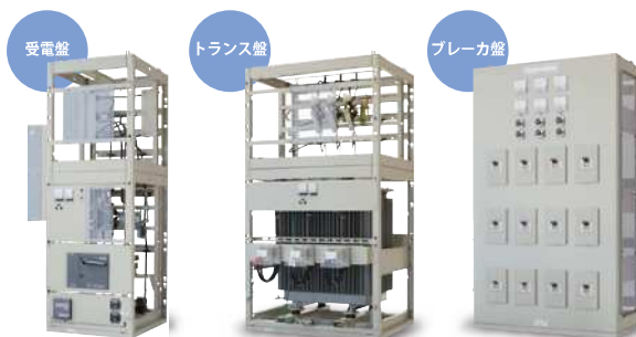
フレーム式高圧受電設備
